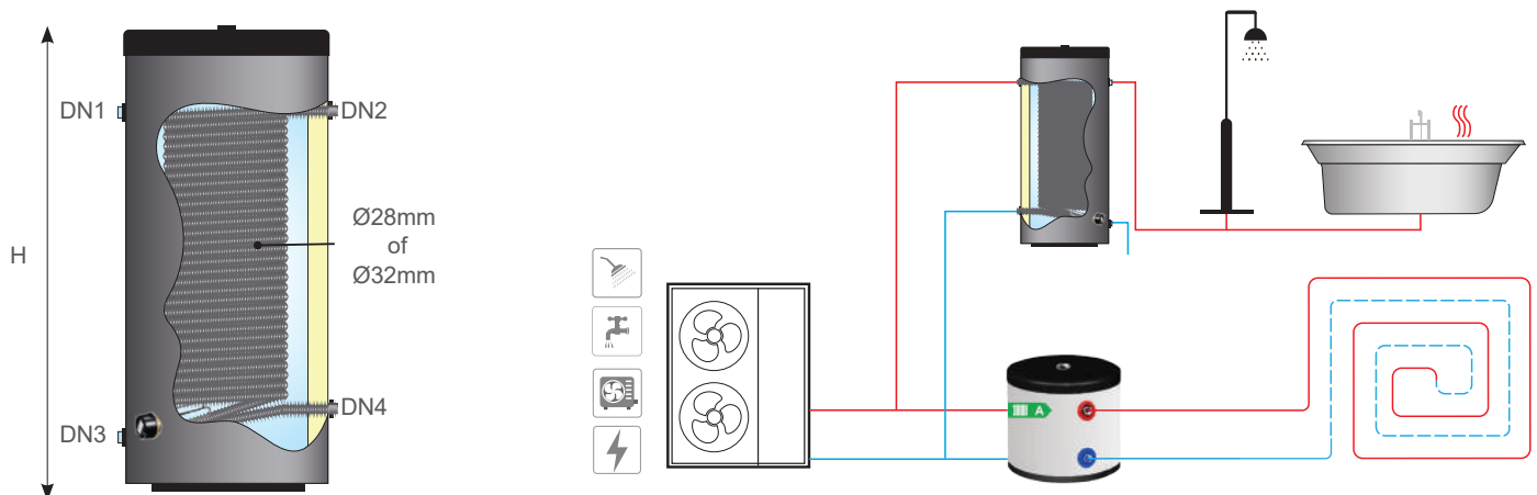
WARMWATERBOILERS MET 1 SPIRAAL - VERTICAAL
