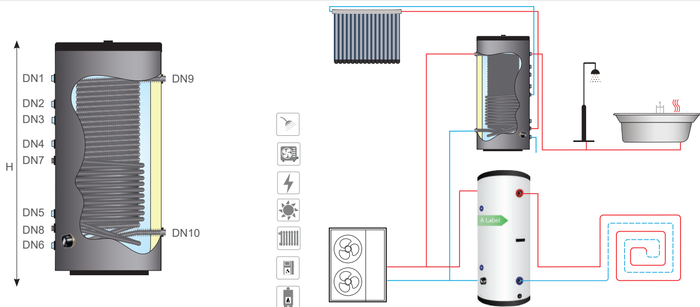
WARMWATERBOILERS MET 2 SPIRALEN VOOR 2 OF MEER WARMTEBRONNEN
