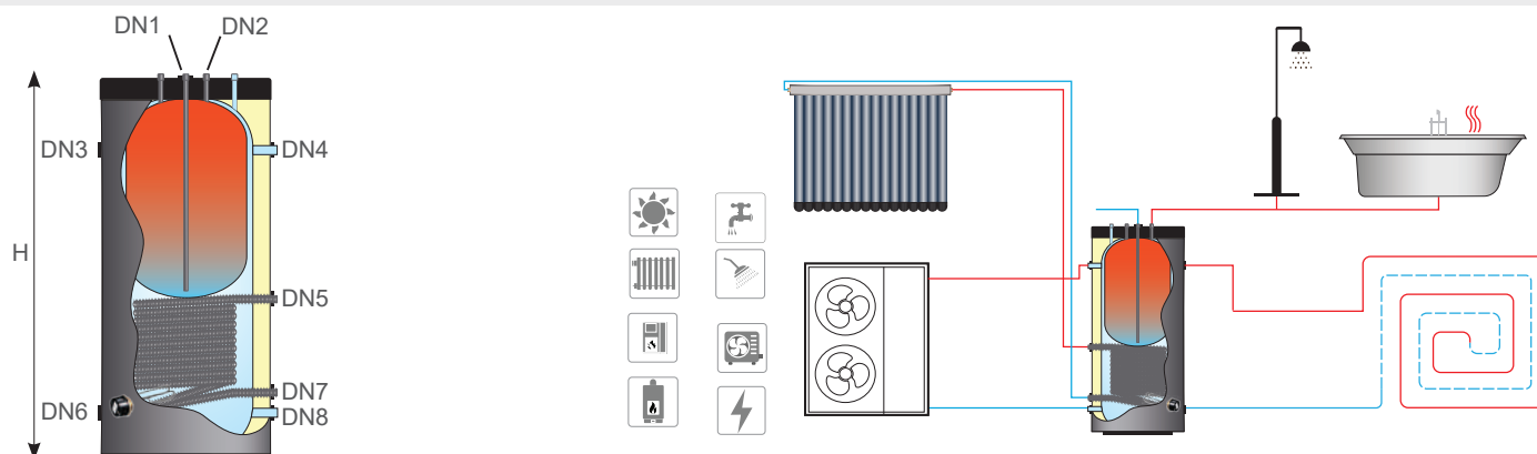
GECOMBINEERDE DOUCHEWATERVERWARMING BINNENIN DE BUFFER
