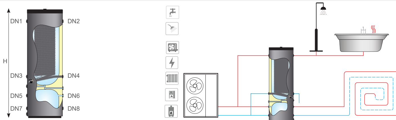
GECOMBINEERDE WARMEPOMPBUFFER EN WARMWATERBOILER
