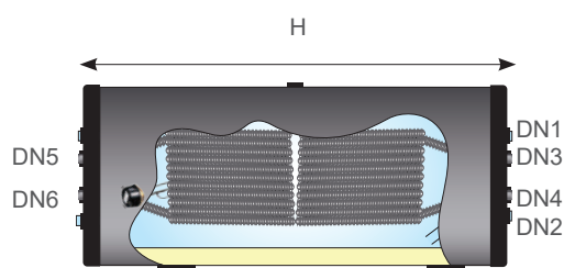
WARMWATERBOILERS MET 2 SPIRALEN VOOR 2 OF MEER WARMTEBRONNEN - HORIZONTAAL
