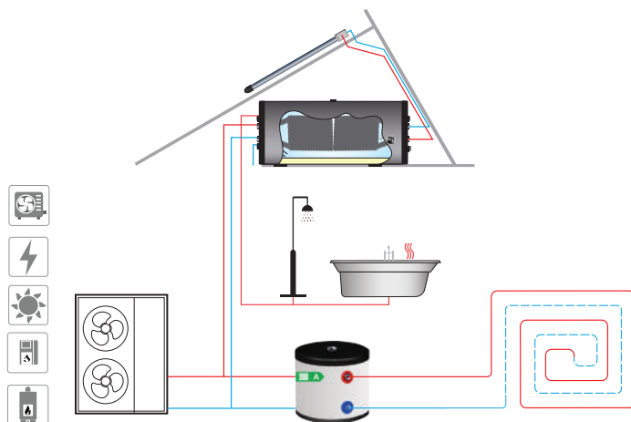
WARMWATERBOILERS MET 2 SPIRALEN VOOR 2 OF MEER WARMTEBRONNEN - HORIZONTAAL
