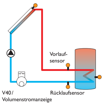
Beispiel für die Positionierung der Vor- und Rücklaufsensoren bei der Wärmemengenzählung.
