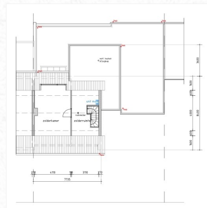
Fig 3. 1ste Verdieping
